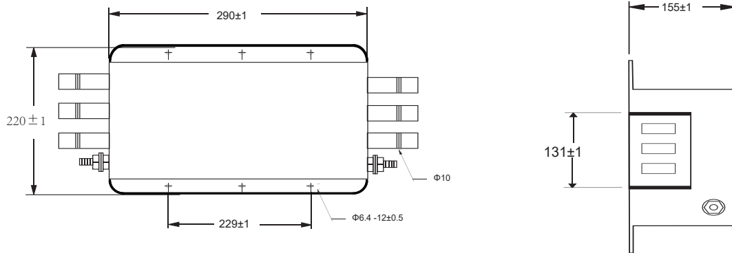
3XBET 外壳样式：3XBET Case Styles
