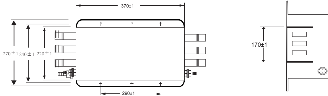
3XBET-B 外壳样式：3XBET -B Case Styles
